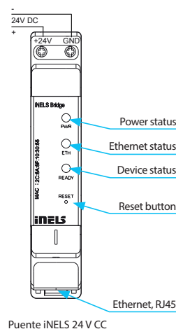
Puente iNELS 24 V CC
